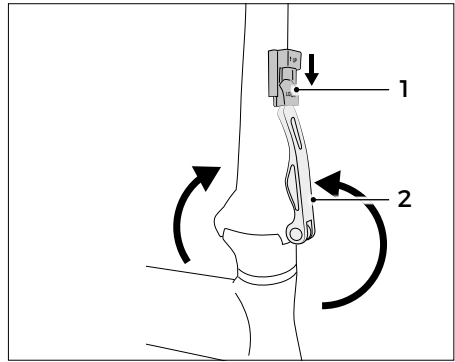
Abb.: Lenkervorbau hochklappen
