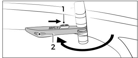
Abb.: Faltscharnier schließen
