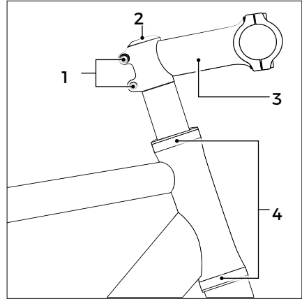
Abb.: Steuerkopfrohr
