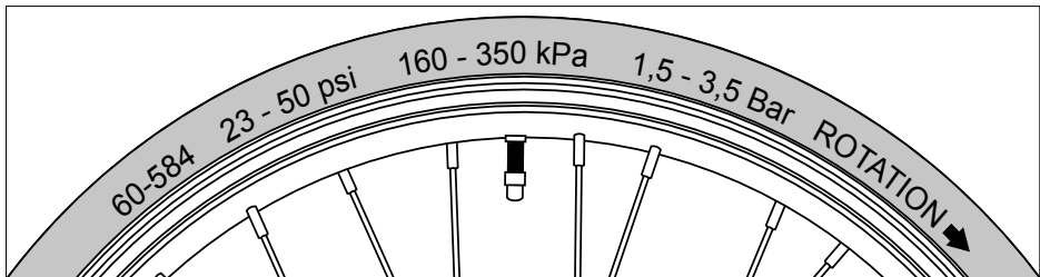
Abb.: Aufdruck auf der Reifenflanke
