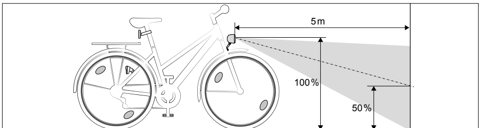
Abb.: Leuchtweite
