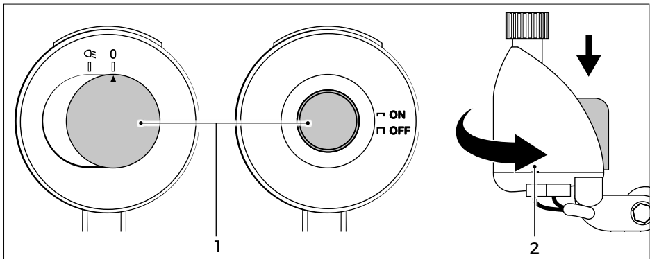
Abb.: Ein-/Ausschalter
