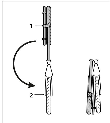
Abb.: Rahmen zusammenfalten
