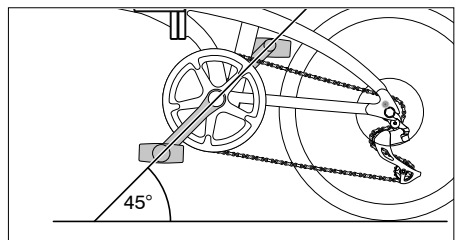
Abb.: Pedaltrieb ausrichten
