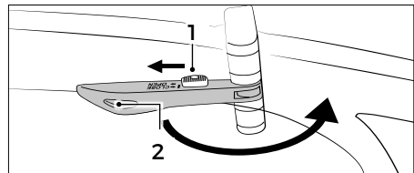
Abb.: Faltscharnier öffnen 1 Verriegelung 2 Spannhebel
