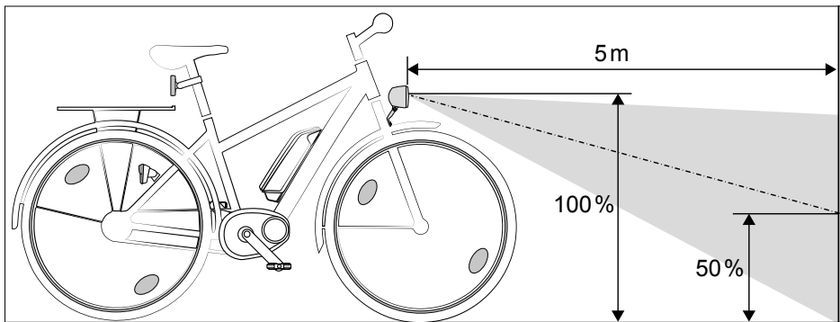
Abb.: Leuchtweite
